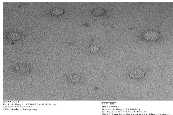
Figure 4a: TEM
